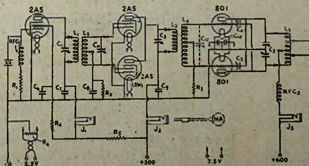
Fig. 1. Het zendschema
