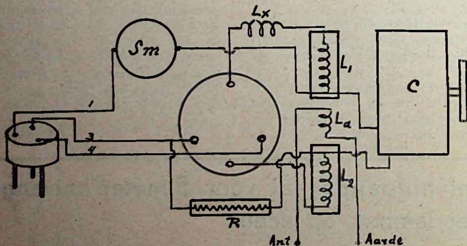
Fig. 2. Het 5 m hulpapparaat voor acculamp bij accutoestel
